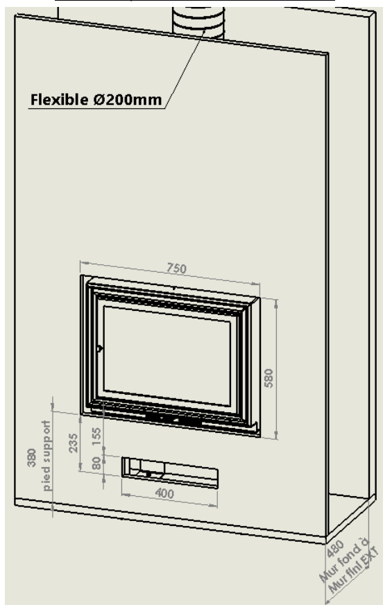
Vue oblique sans cadre de finition
